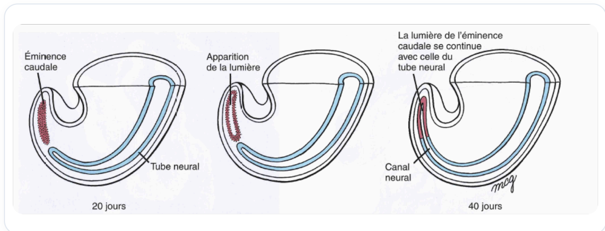
ABB. — Entwicklung der Eminentie/des Neuralkanals
